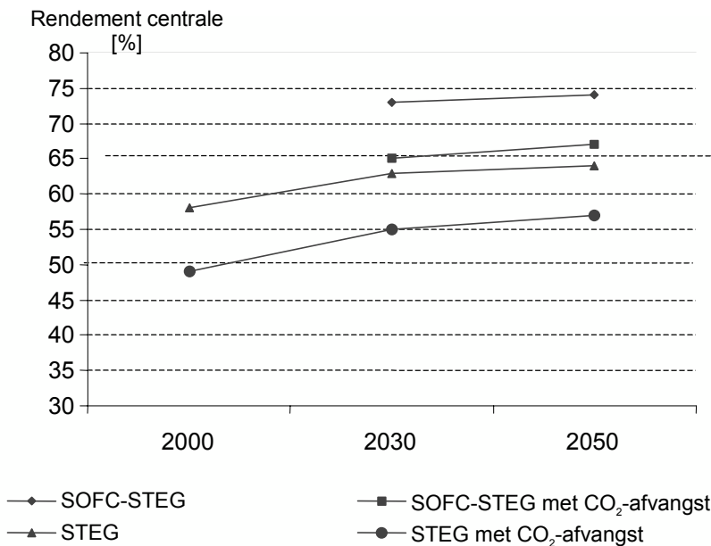
Figuur 2.1 Verwachte ontwikkeling rendement gasgestookte elektriciteitsopwekking
